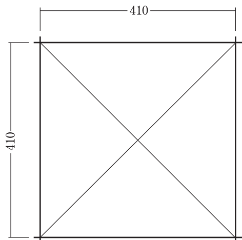
図1 開口寸法
